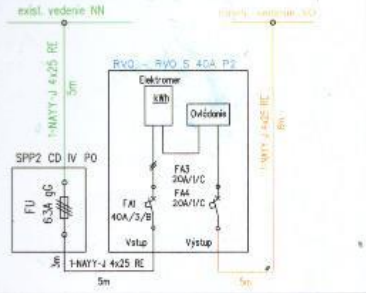
Jednopolová schéma napojenia RVO
