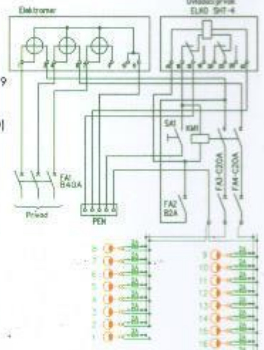
ROZVÁDZAČ VEREJNEHO OSVETLENIA - RVO
